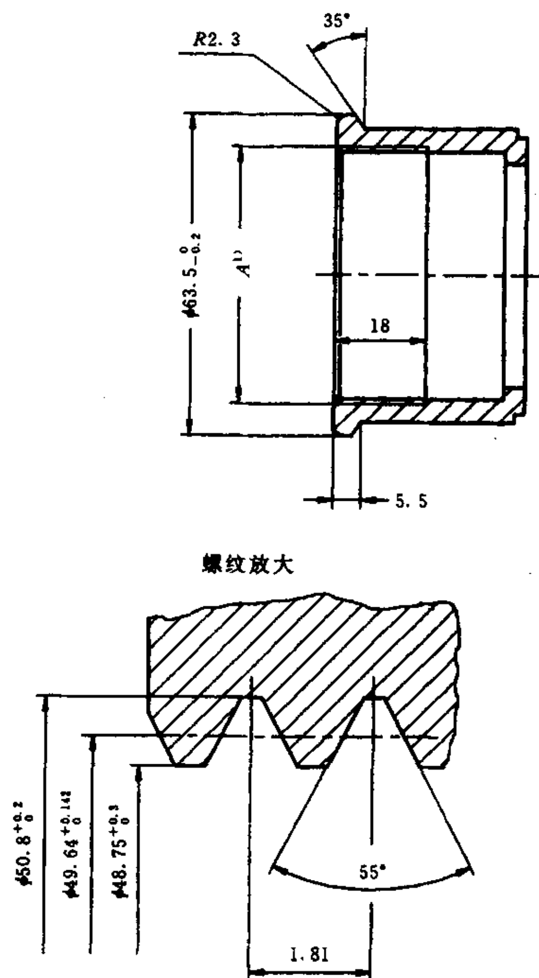
图 B1 连接座外形及连接螺纹尺寸
