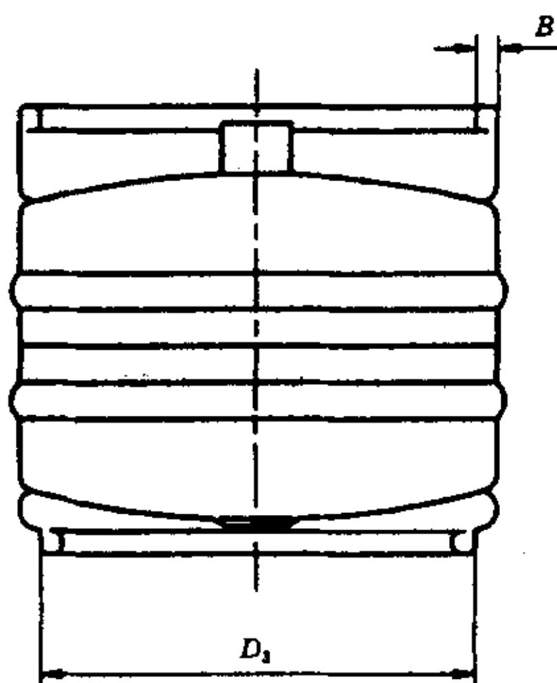
图 A1 啤酒桶止口
